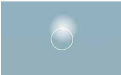
日本各地での欠け方のようす 素材の種類：HD映像 (CG)
