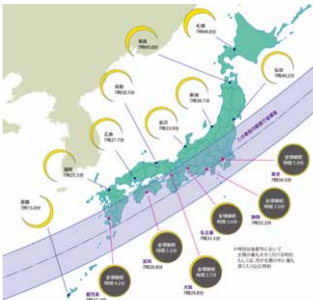
2012年5月21日の日本各地のようす。 (この図版はご提供可能です)
