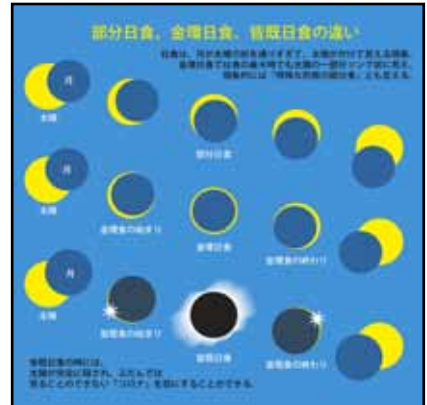
部分、金環、皆既日食の違い 素材の種類：図版
