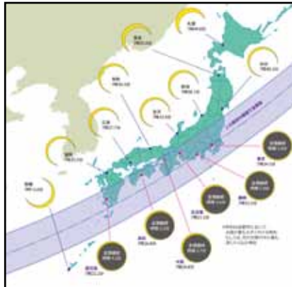
日本各地での欠け方のようす 素材の種類：図版
