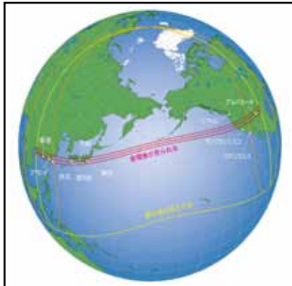
金環・部分日食が見られる範囲 素材の種類：図版
